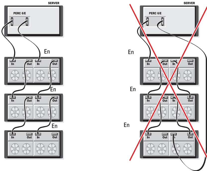
Ilustración 3-13. Configuración del soporte de rutas de acceso redundantes con tres alojamientos
