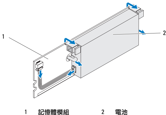
圖 2. 卸下 BBU
